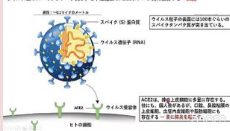
ウイルス上のスパイクタンパク質が、ヒト細胞上のACE2タンパク質に結合する一瞬間
